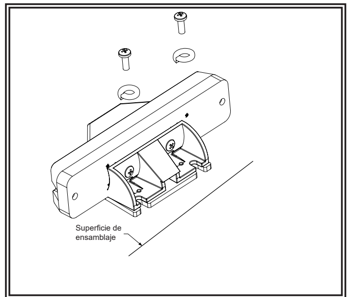
Ensamblaje permanente
