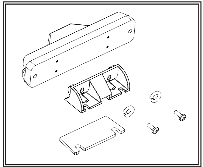
Ensamblaje adhesivo
